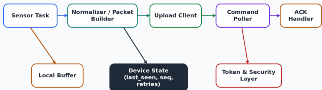
Hình 7.2. Kiến trúc firmware theo mô-đun chức năng trên thiết bị ESP32.
